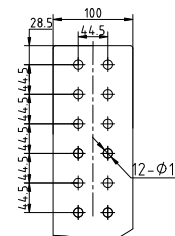
L.V. TERMINAL
